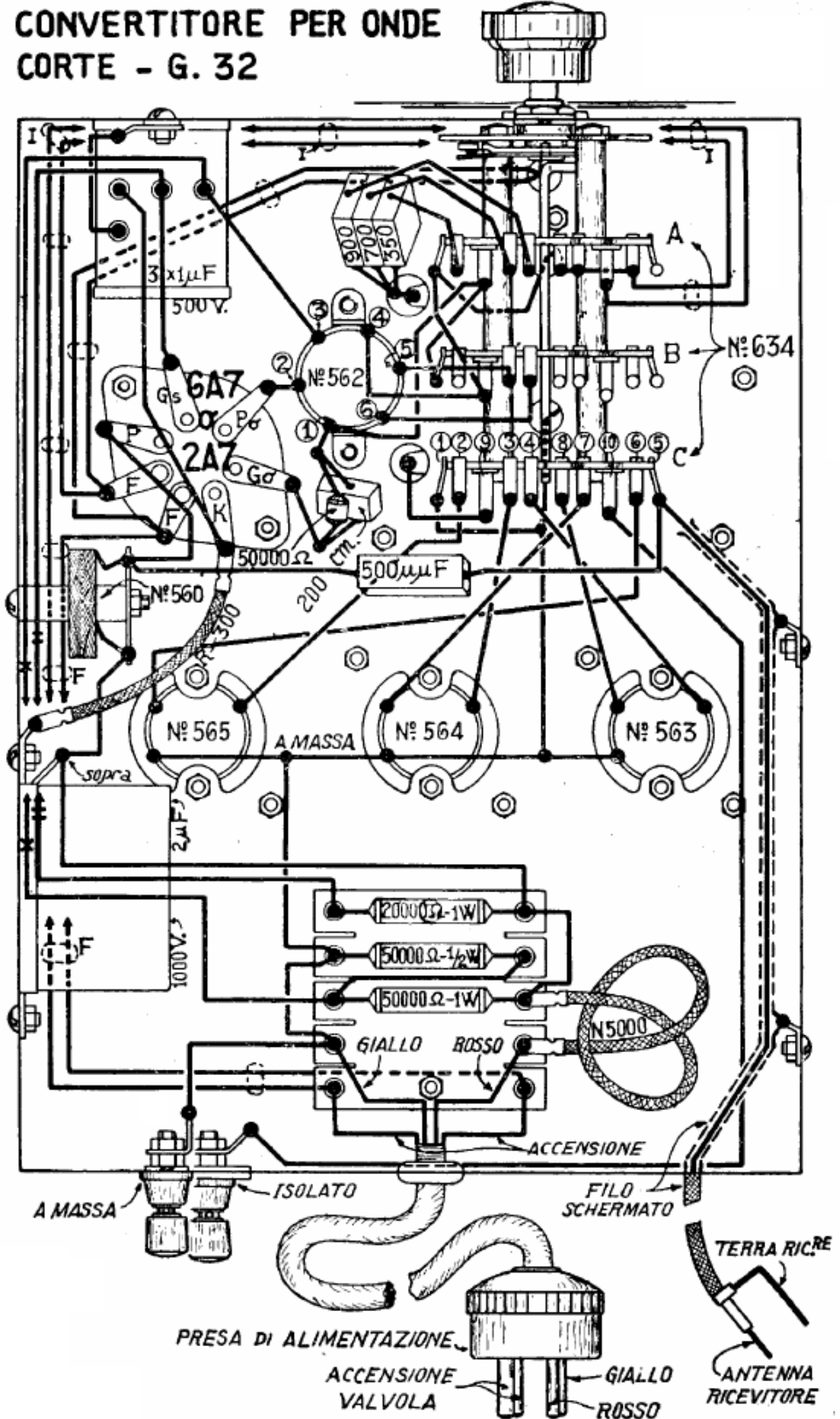
- Schema costruttivo del convertitore per onde corte G-32.
